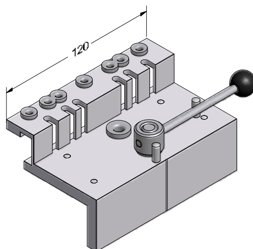
Шаблон для механического соединения, сверления отверстий фиксаторов горбылька 68
